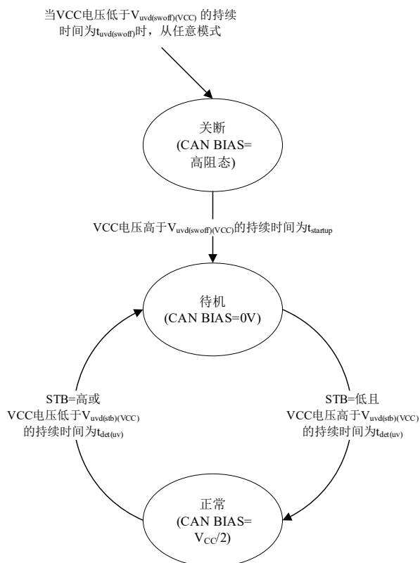
图 9 SIT1044AQ 状态图
