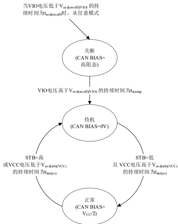
图 8 SIT1044AQ/3 状态图
