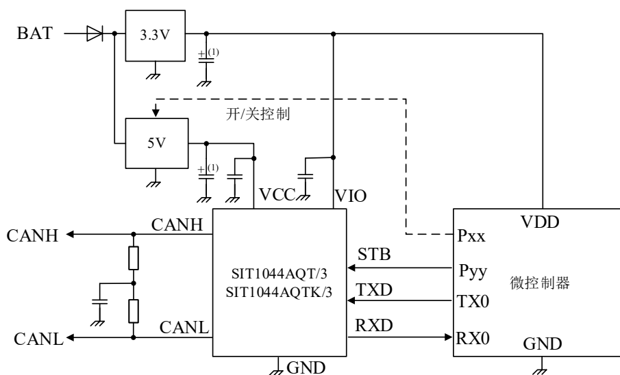
图 6 SIT1044AQ/3 3.3V 微控制器典型应用
