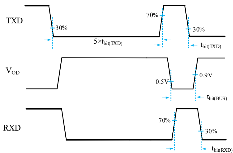
Fig 2 t_{\text{bit}} delay
